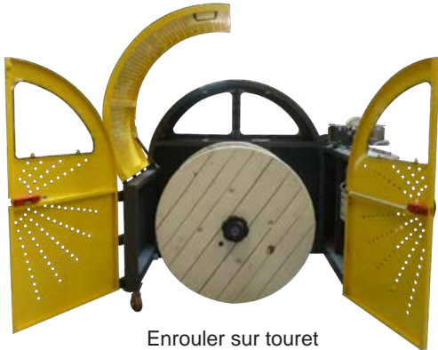
Enrouler sur touret (maxi 400kg et Ø 1050mm)
