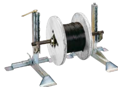
AXO 1600 Vis sans fin
